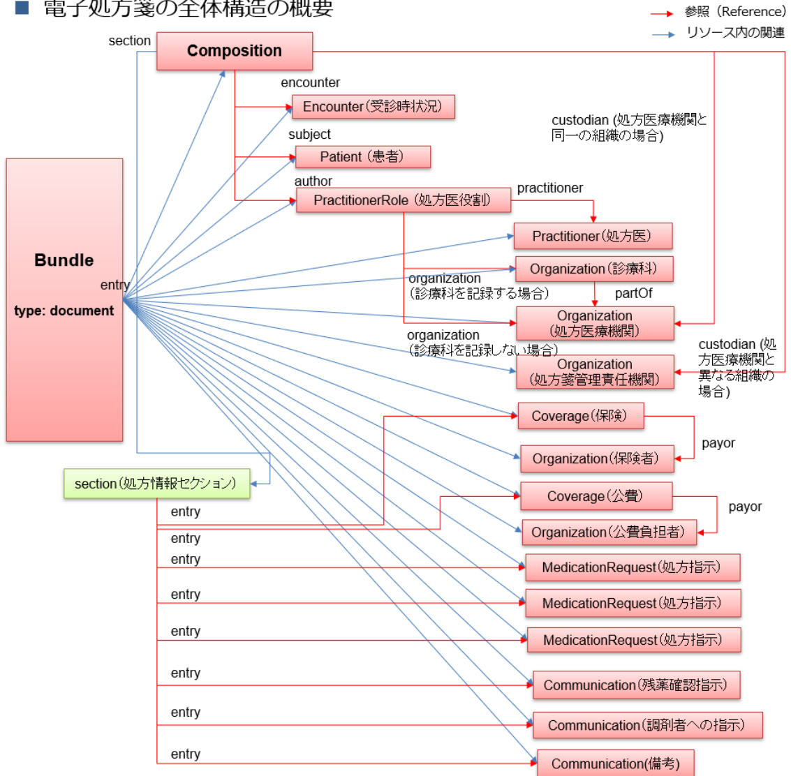
図 3 処方箋データの全体構造の概要
